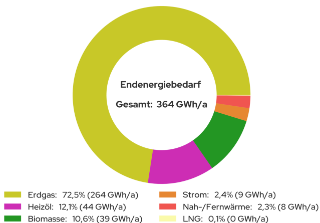
Abbildung 15: Endenergiebedarf nach Energieträger in Mühlacker
