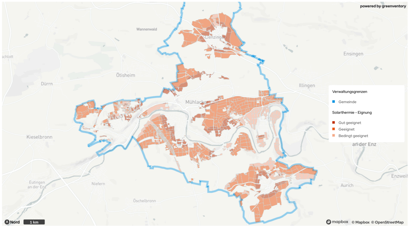
Abbildung 40: Nutzbare Wärmeenergie aus Sonnenstrahlung
